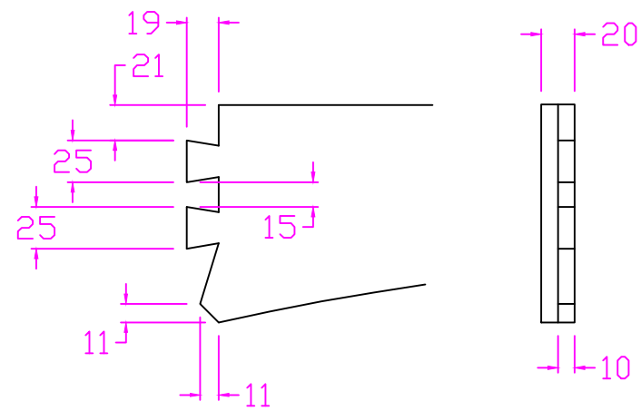
FRONT RAIL - HALF LAP DOVETAILS TRAVERSE AVANT - ASSEMBLAGE A QUEUE D'HIRONDE a MI-BOIS
